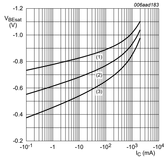
I_C/I_B = 20 (1) T_{amb} = -55 °C (2) T_{amb} = 25 °C (3) T_{amb} = 100 °C
